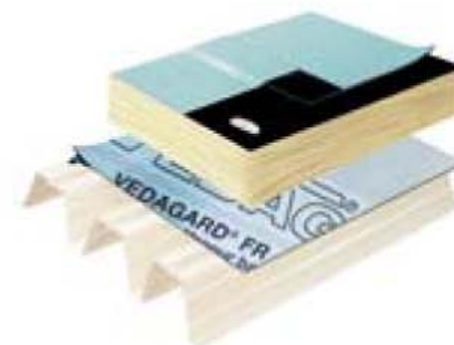
VEDAPROOF® TV Industriedach nach DIN 18234
