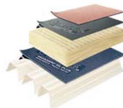
VEDAG ProfiDach Mineralwolle auf Profiblech
